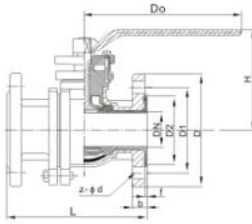
衬氟O型球阀(Q41F46)
